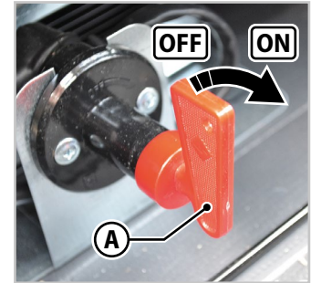
Abb.6.30 - Batterietrennschalter
