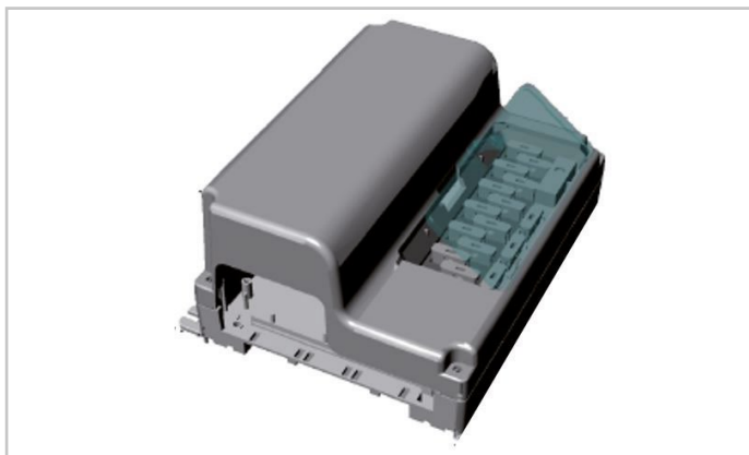
Abb.7.2 - Sicherungshalter C/Poliswitch
