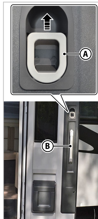
Abb.5.2 - Öffnen/Schließen der Eingangstür von innen
