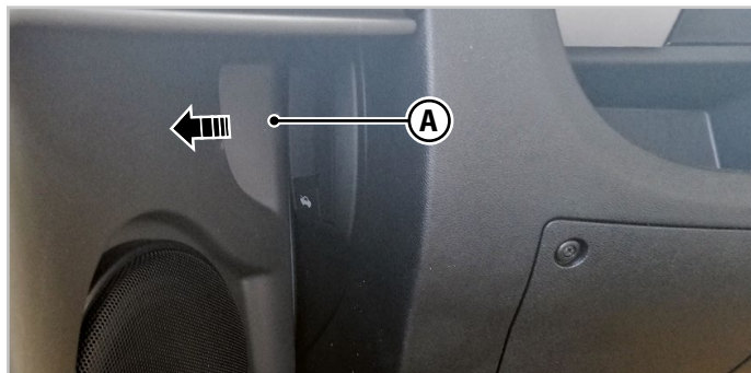
Fig.5.8 - Palanca de apertura del capó - Tipo A
